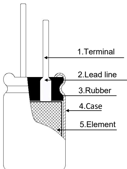
Capacitor 电容器
